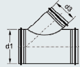
Trójnik 45° BDEV-1
