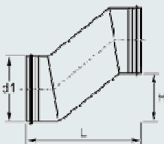
Odsadzka ETES-1
