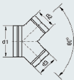
Trójkąt orłowy BDOY-1
