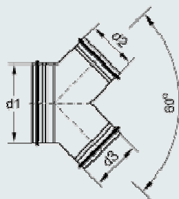
Trójnik orkowy BDEY-1
