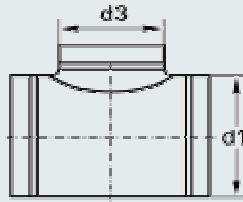
Trójnik 90° BDOT-1
