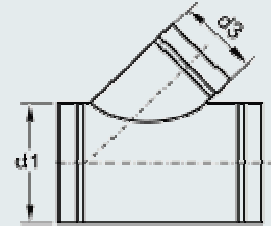
Trójnik 45° BDOV-1
