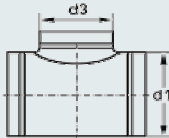
Trójnik 90° BDOT-1
