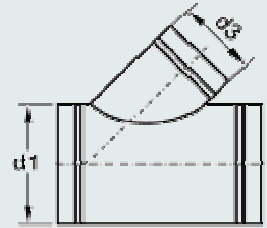
Trójnik 45° BDOV-1
