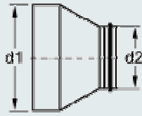
BDEF-1 zew/wew
