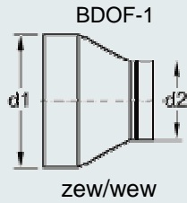
Zwężka symetryczna
