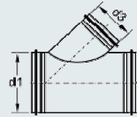
Trójnik 45° BDEV-1
